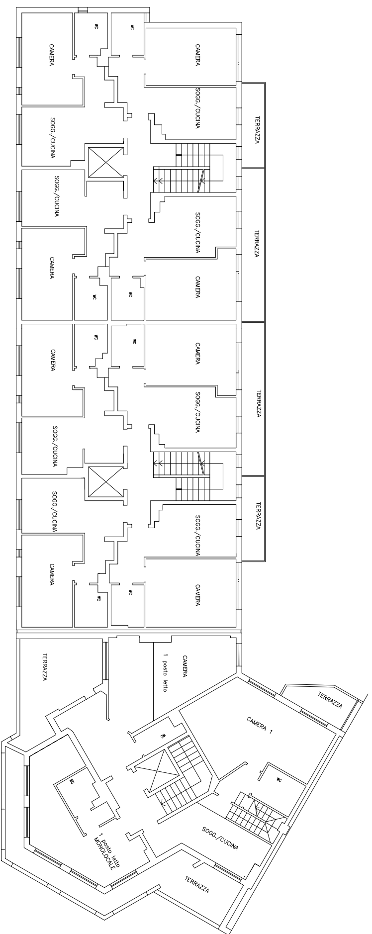
PIANTA PIANO QUARTO
