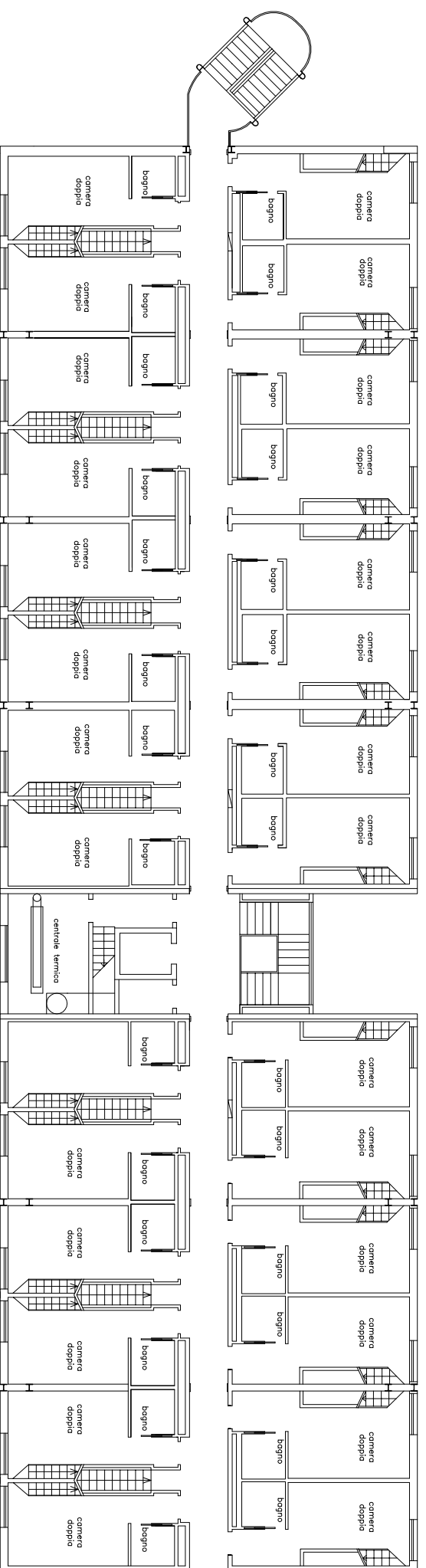
PIANO SECONDO
