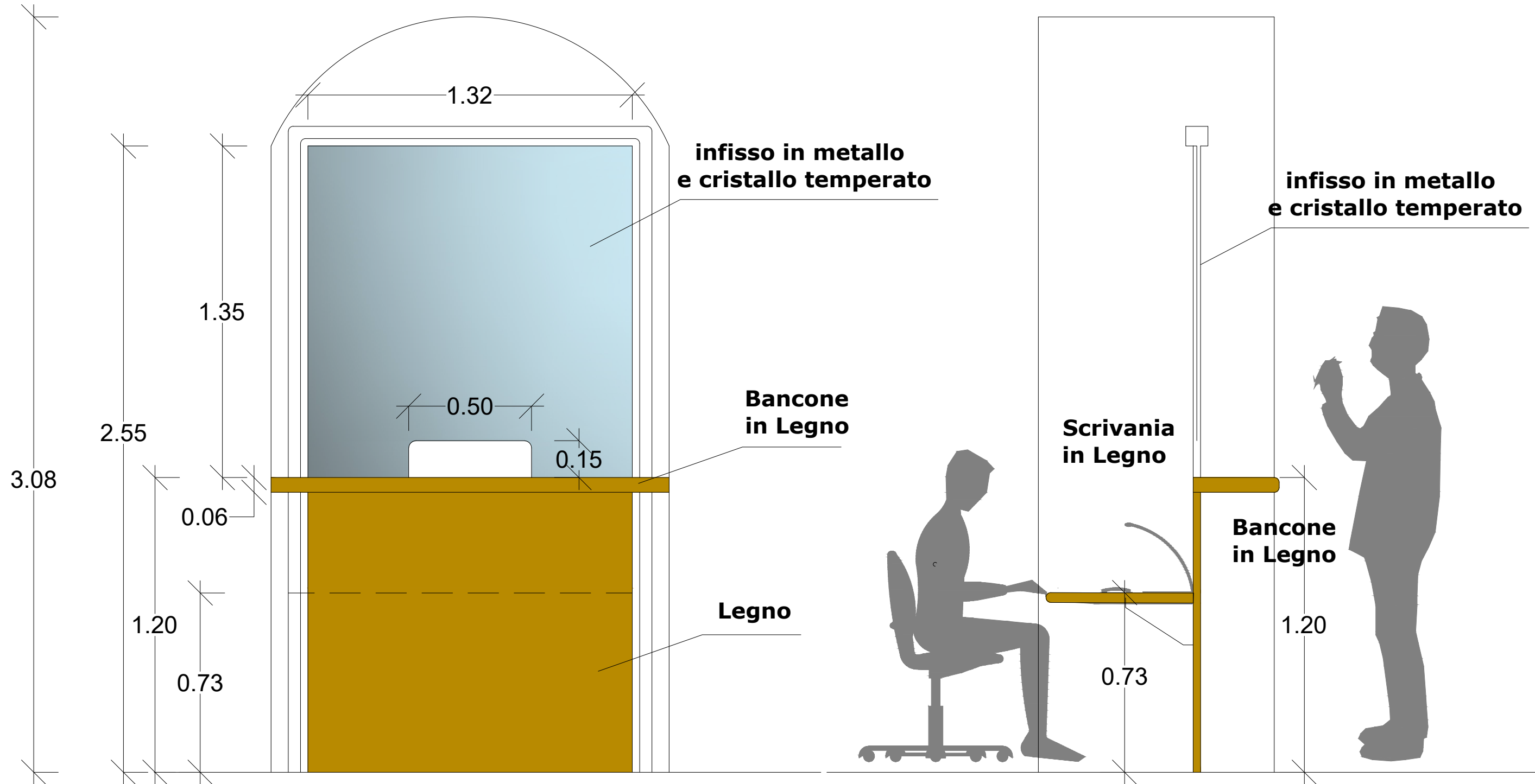
PROSPETTO FRONT OFFICE
